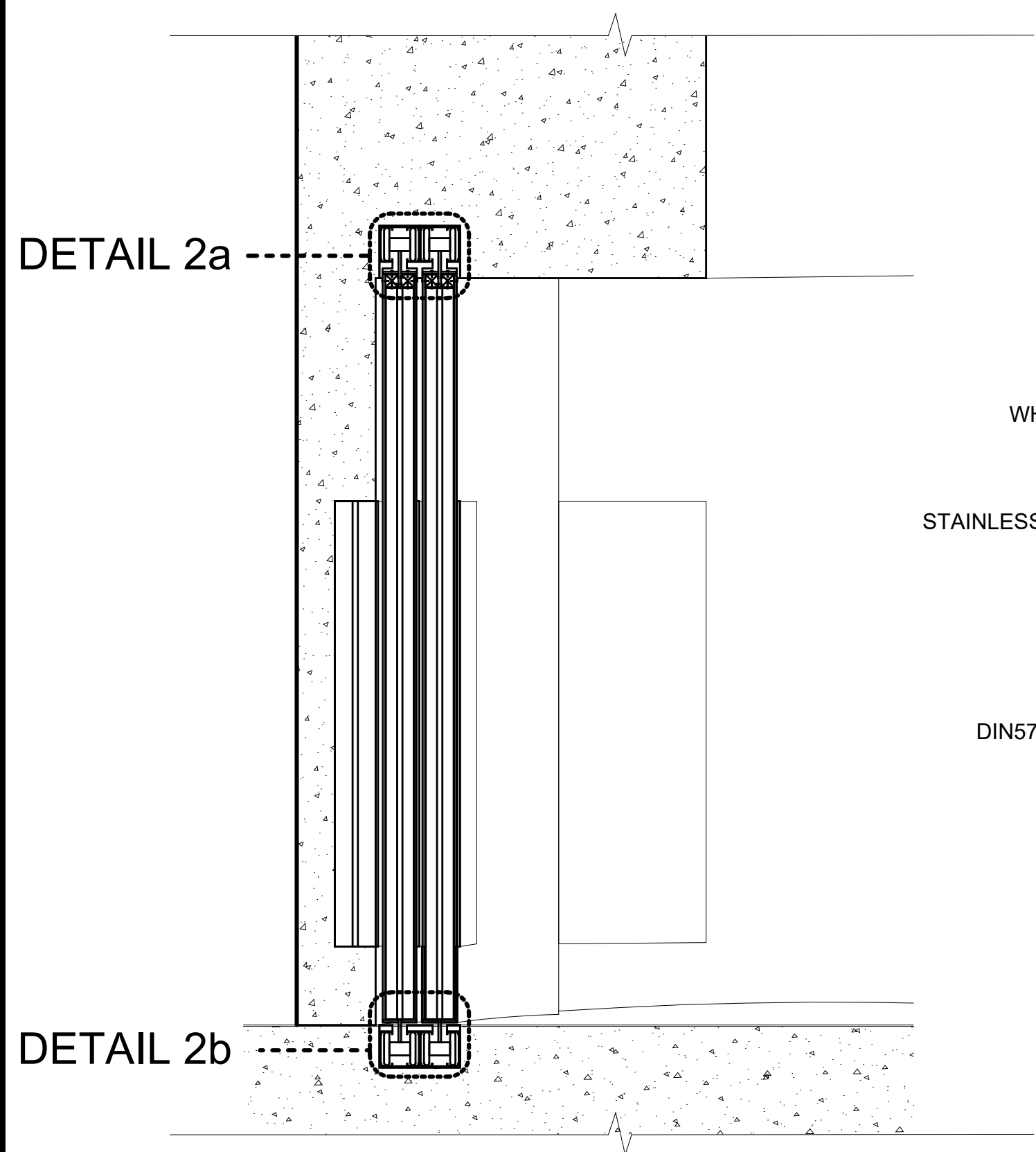
3 602 DETAIL 2: SECTION A-A SCALE : 1 : 20
