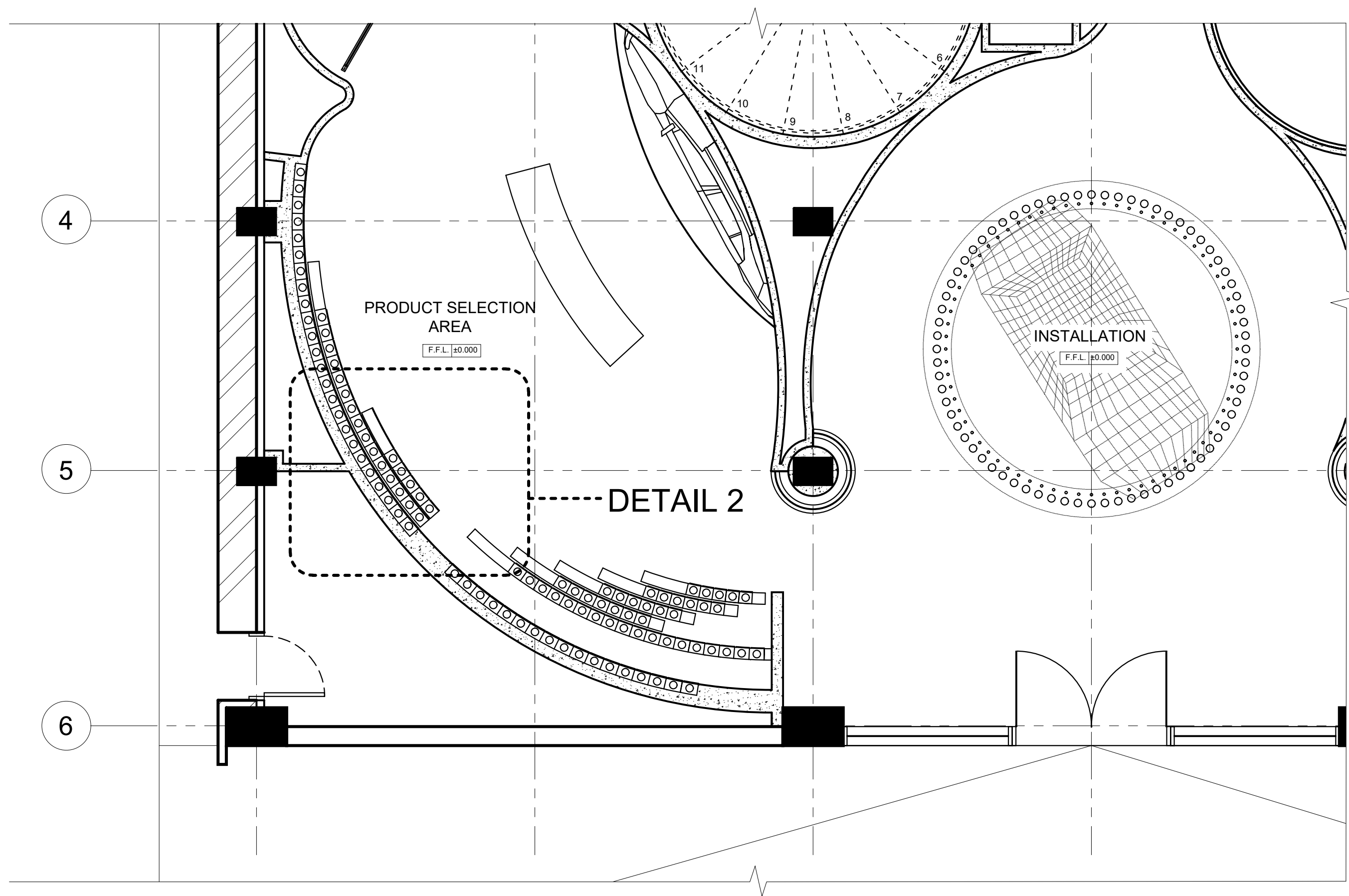
1 602 KEY PLAN SCALE : 1 : 50
