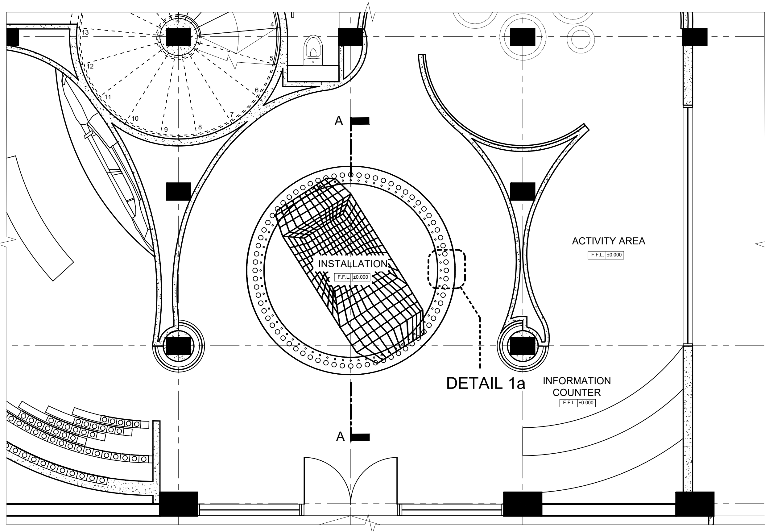
1 601 KEY PLAN SCALE : 1 : 50
