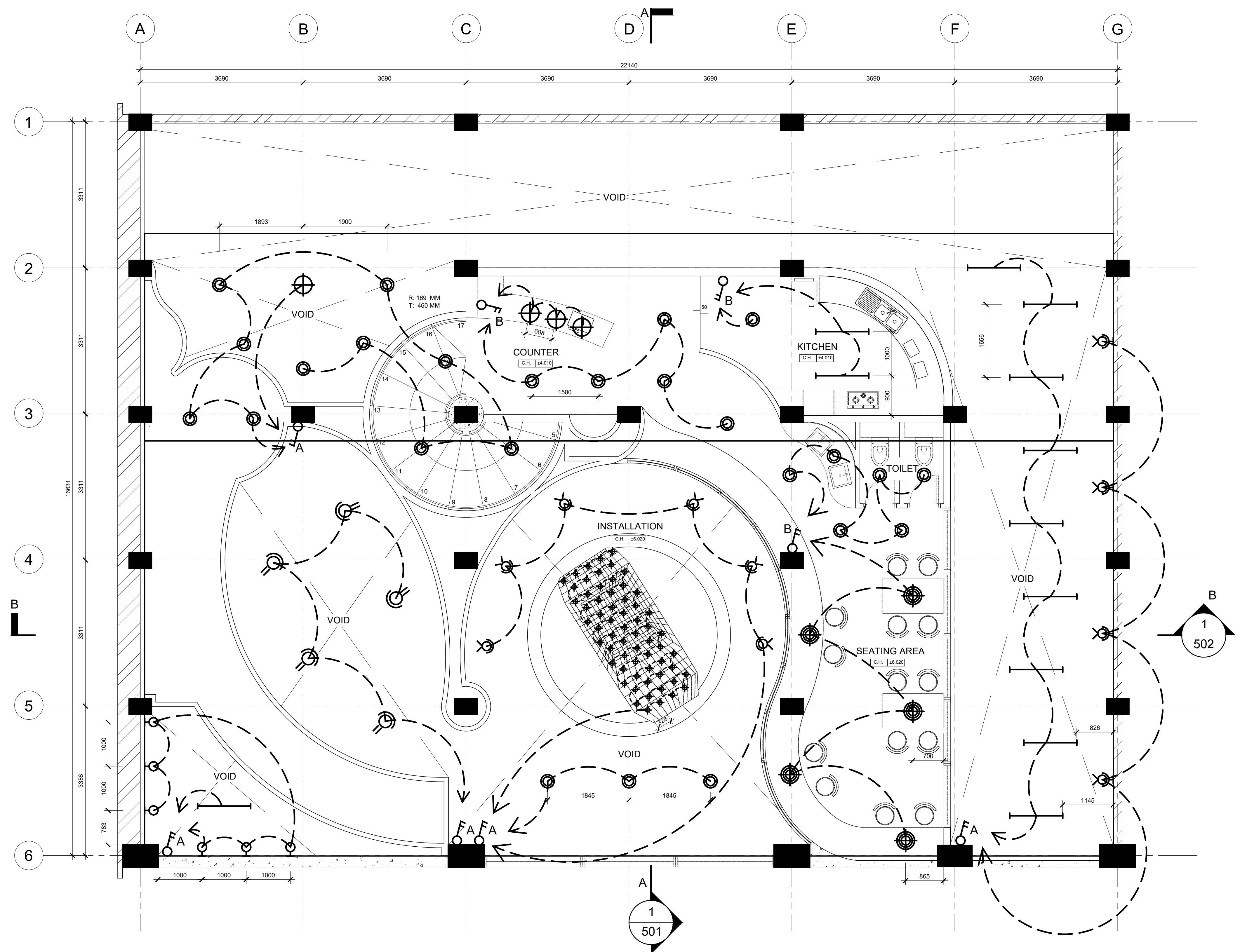
1 202 RCP - LEVEL 2 SCALE : 1 : 50
