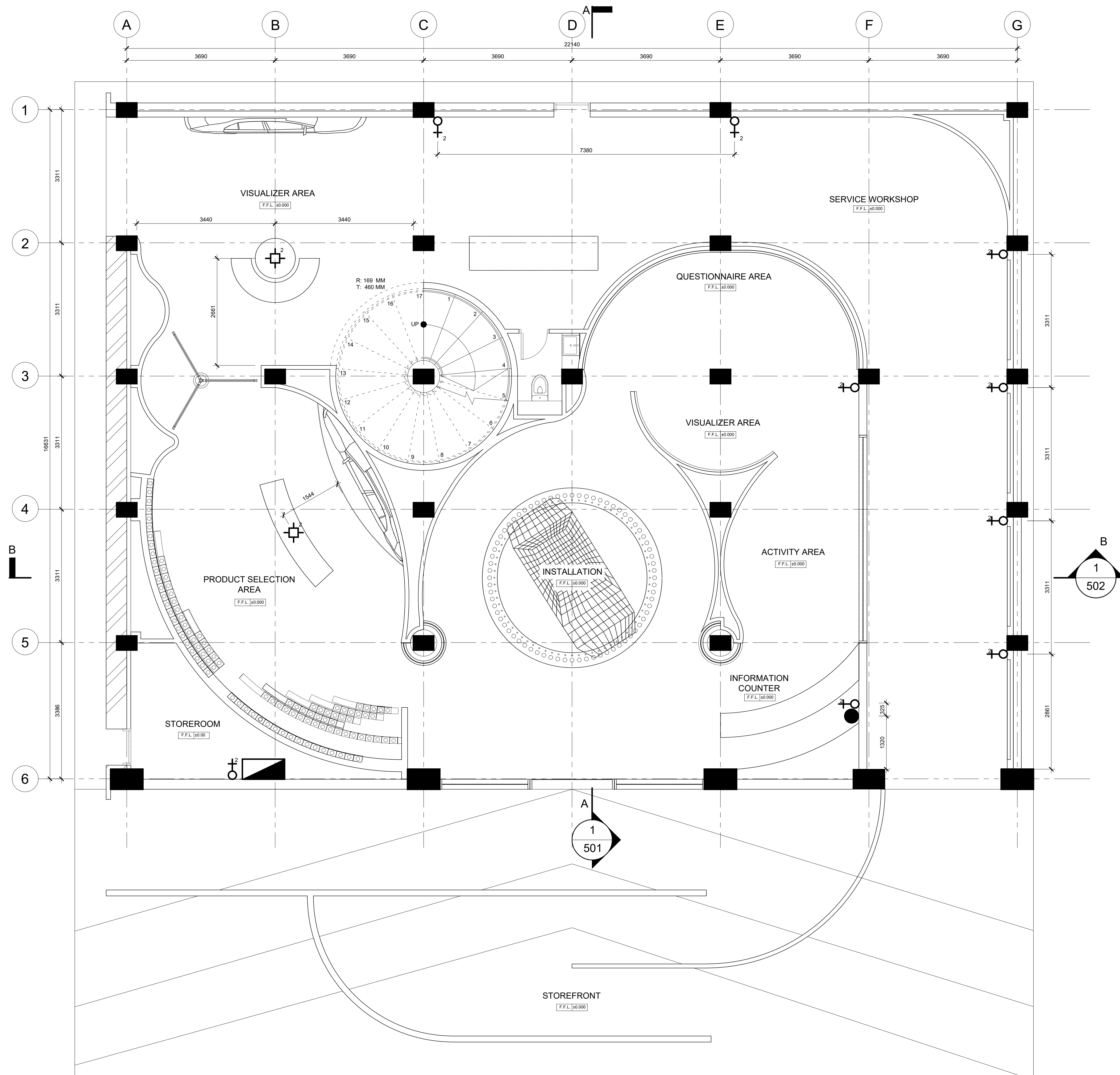
ELECTRICAL & DATA PLAN - LEVEL 1 SCALE : 1 : 50
