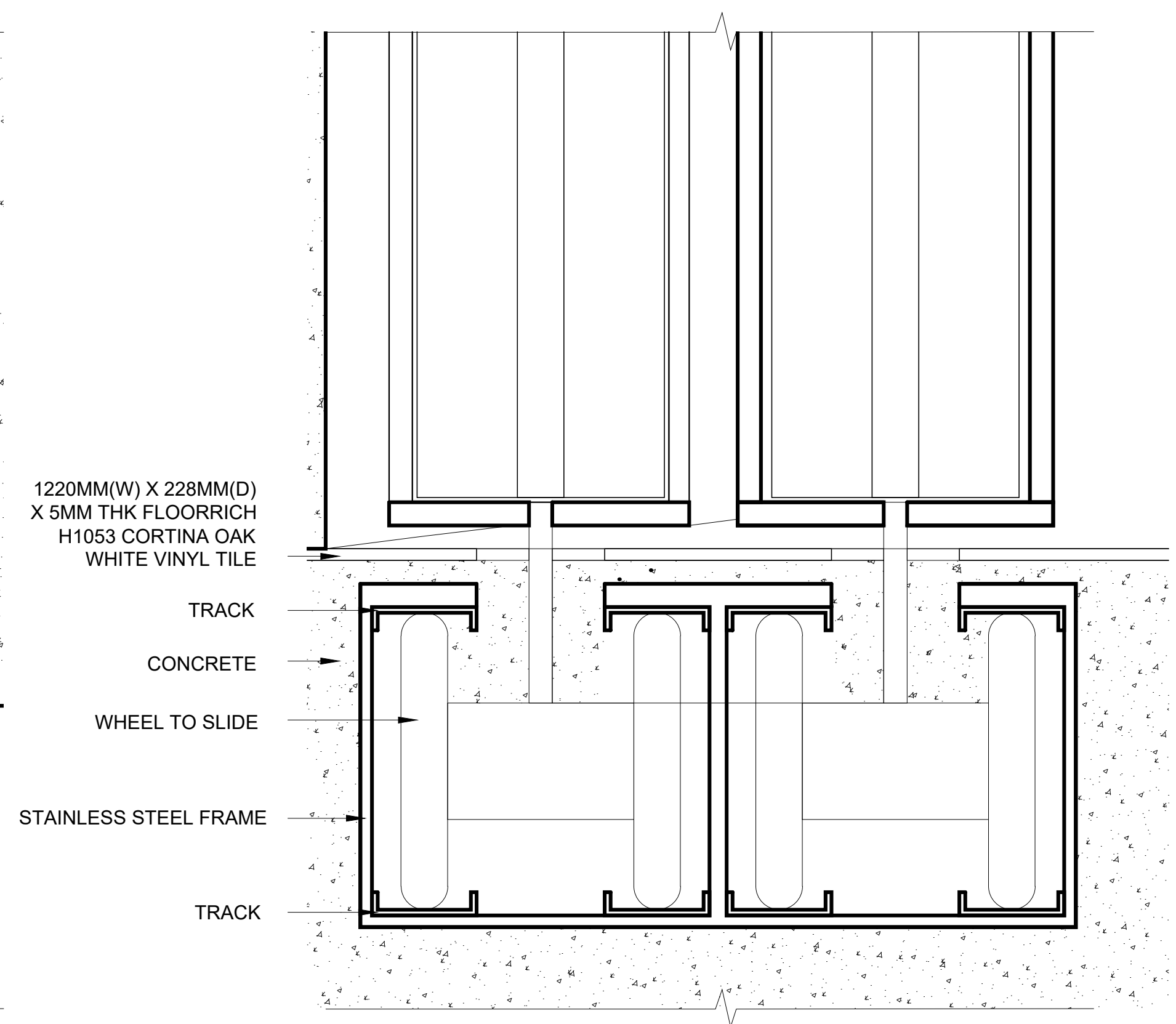
5 602 DETAIL 2b SCALE : 1 : 2
