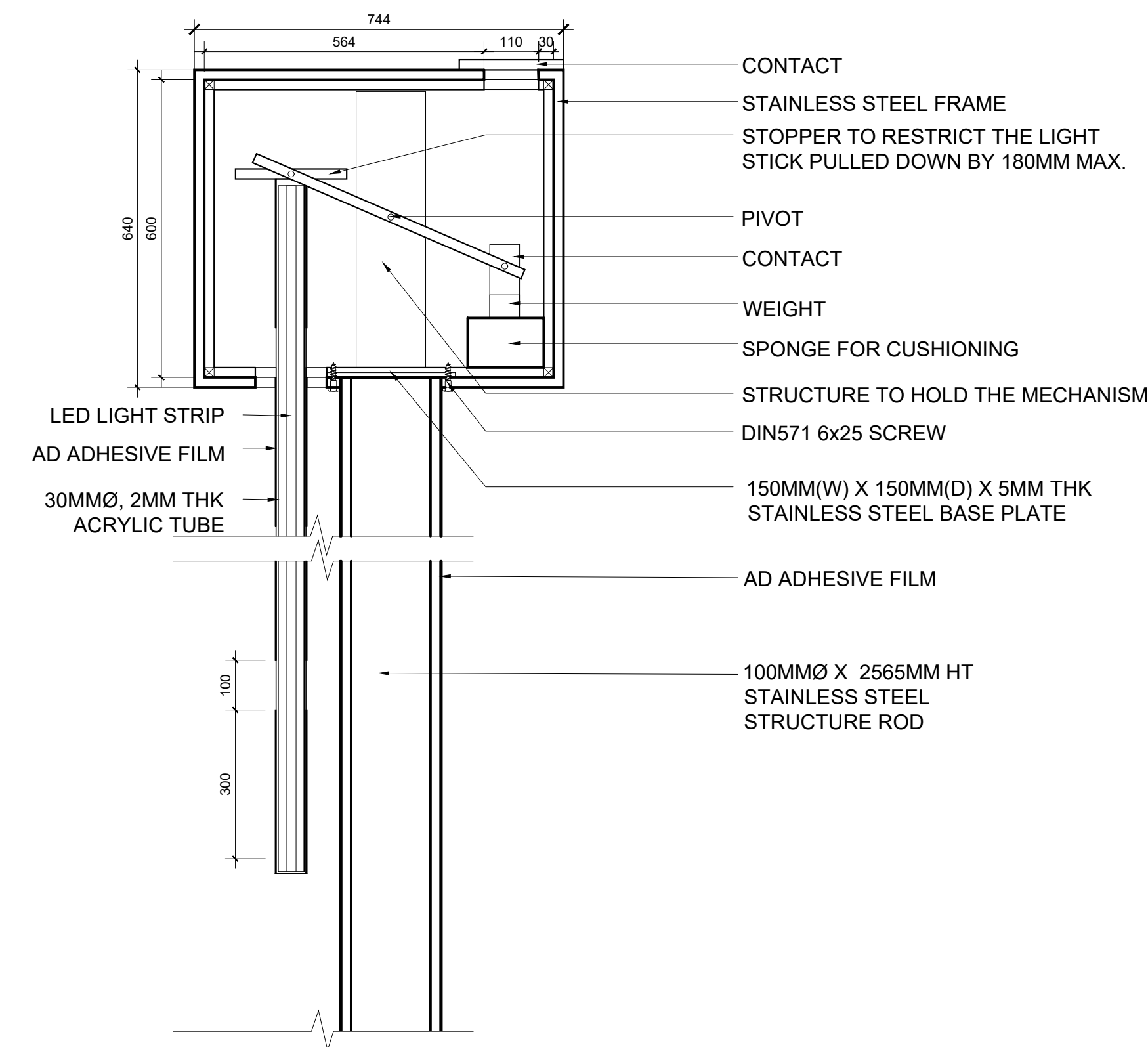
3 601 DETAIL 1a: SECTION B-B SCALE : 1 : 5
