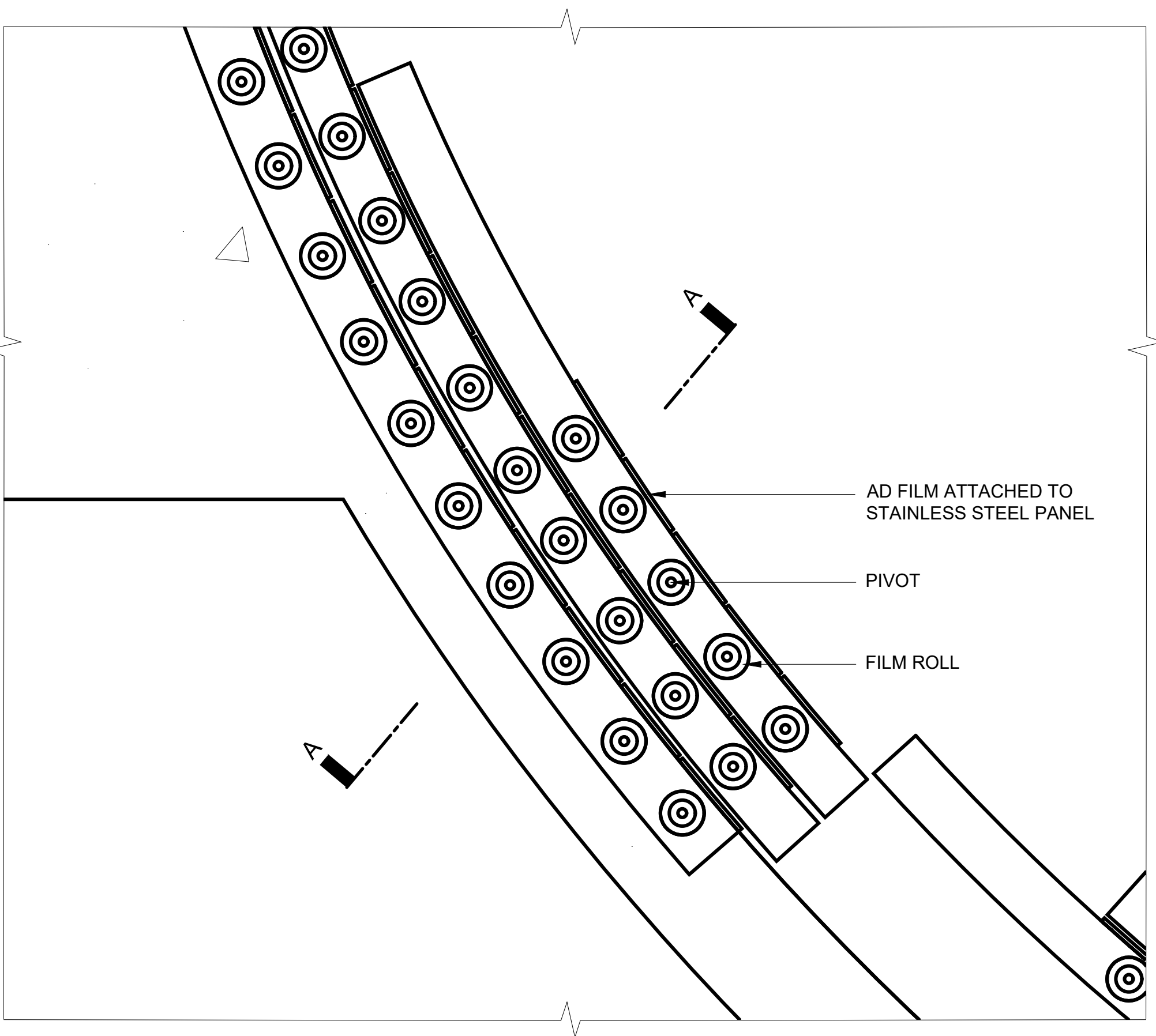
2 602 DETAIL 2: PLAN SCALE : 1 : 25
