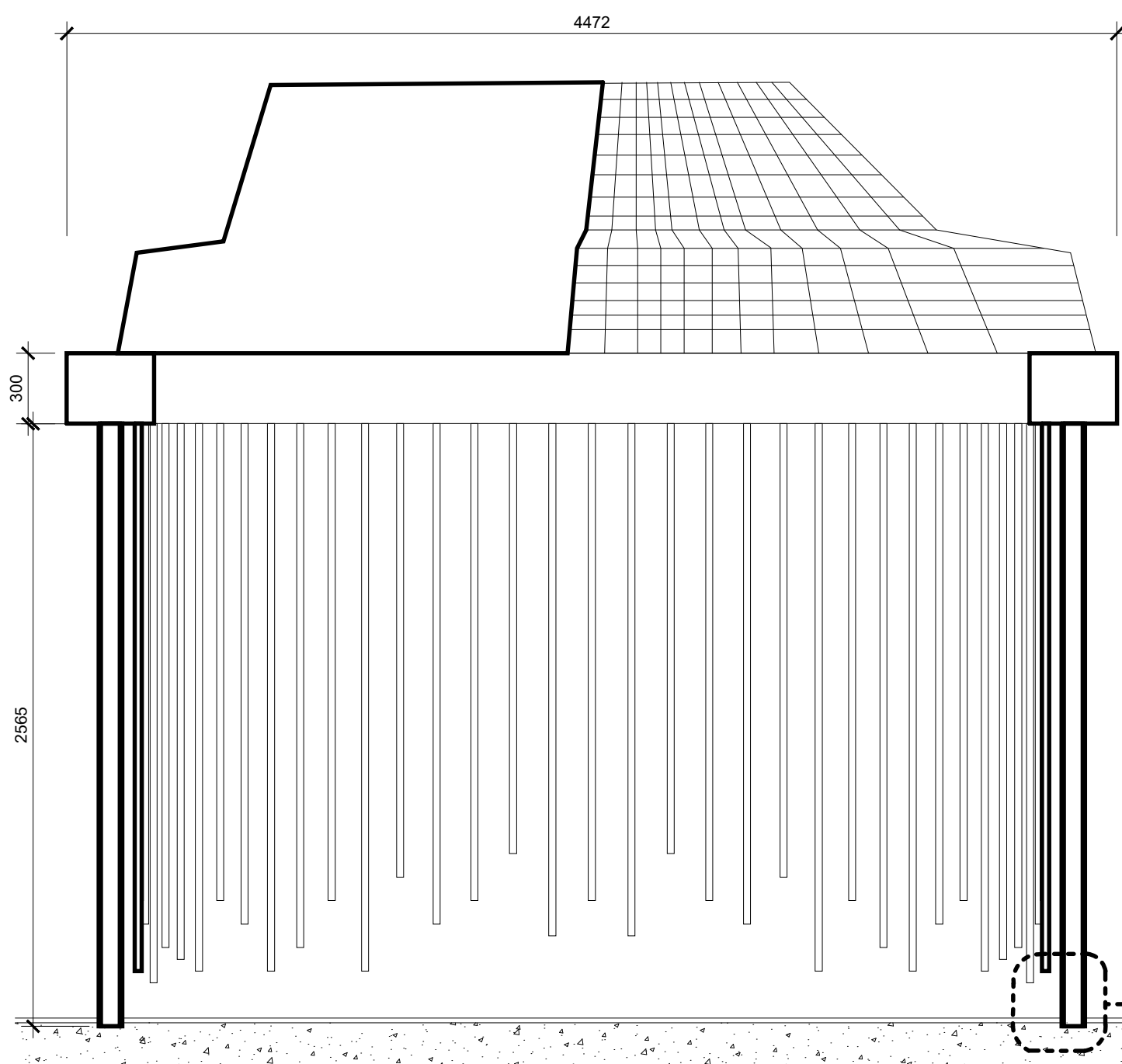
4 601 SECTION A-A SCALE : 1 : 50
