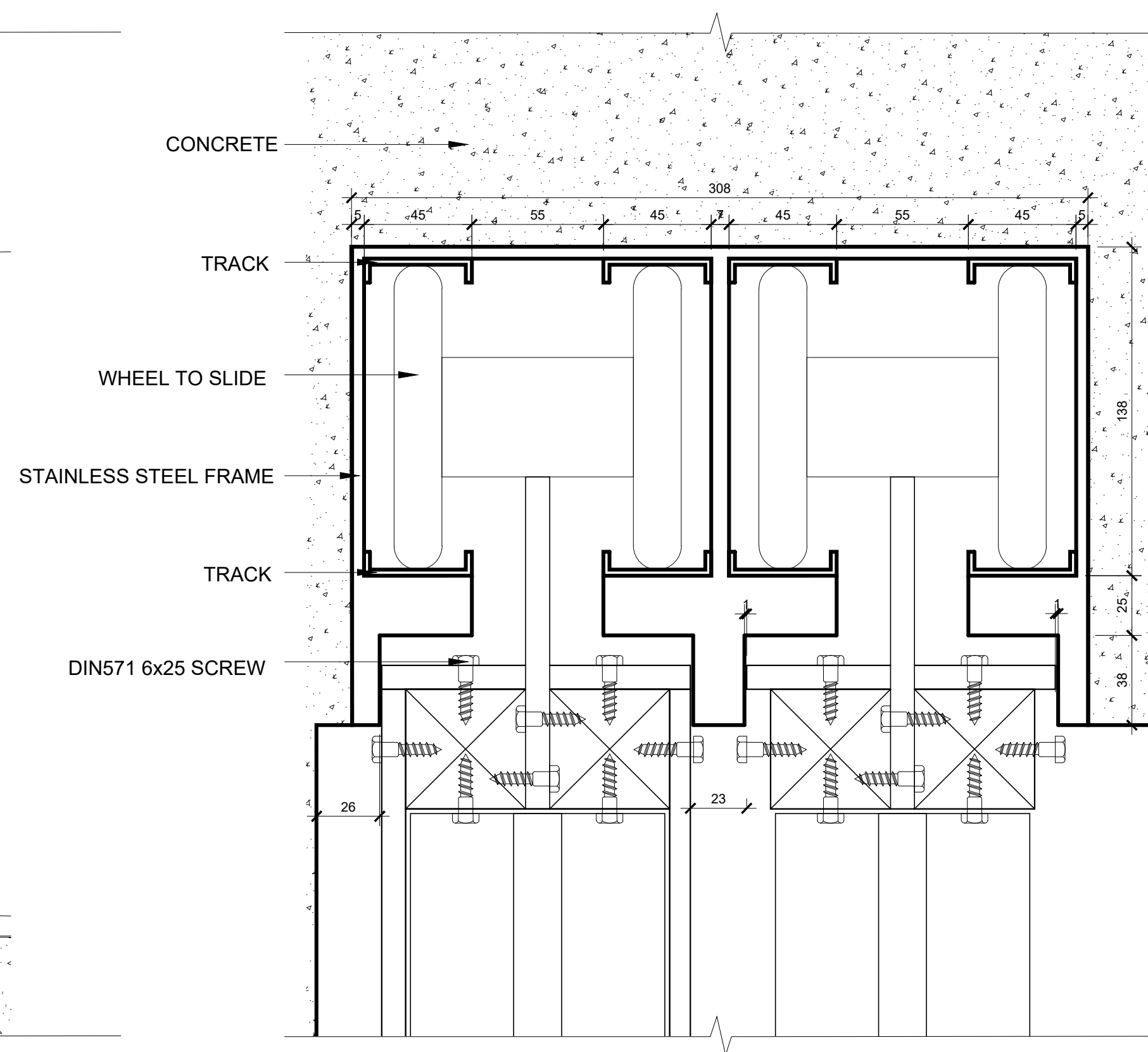
4 602 DETAIL 2a SCALE : 1 : 2
